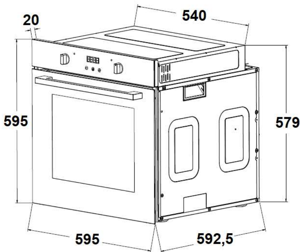
ABB. 1: MAßE / BACKOFEN
