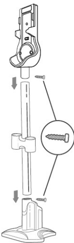
Support de charge avec deux vis
