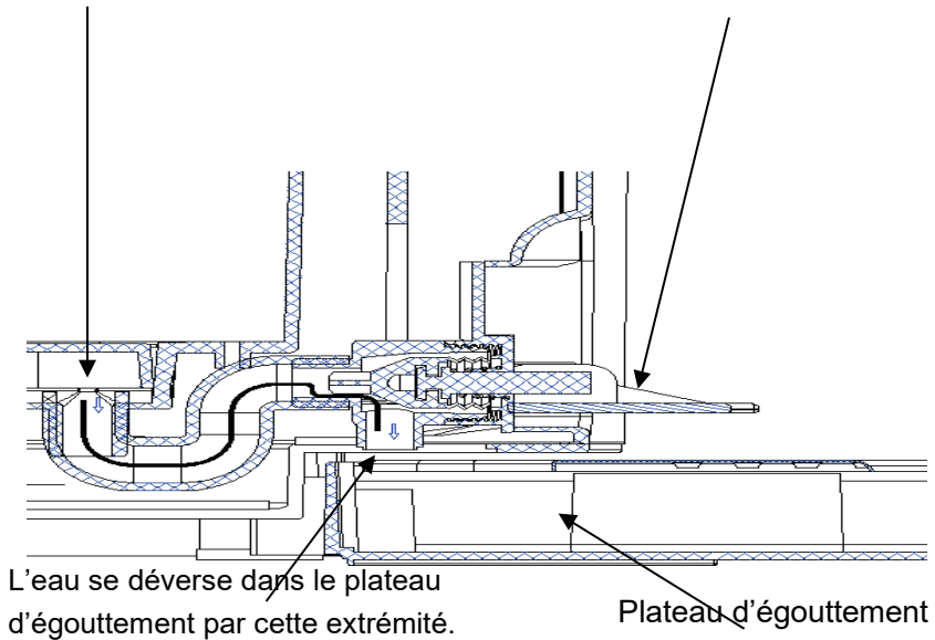
Figure 15 (schéma du circuit de vidage)
