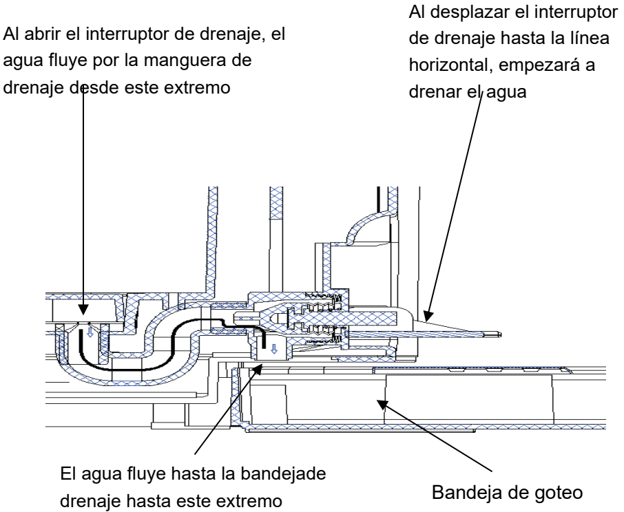
Figura 15 (Esquema del sistema de drenaje)
