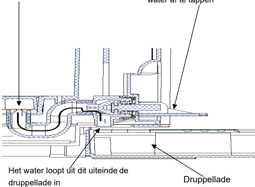
Figuur 15 (afbeelding van drainagestructuur)
