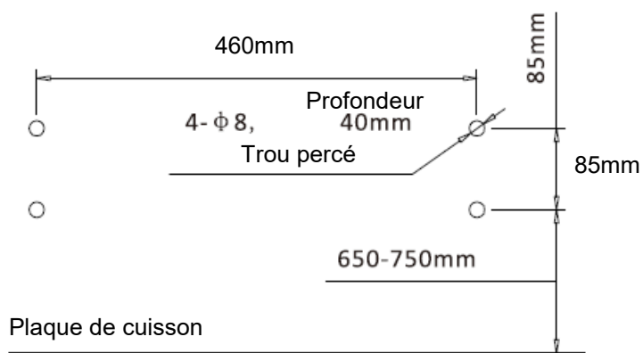
Schéma représentant la taille des trous à percer
